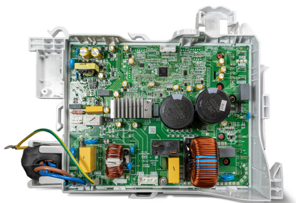
Tarjeta condensadora
